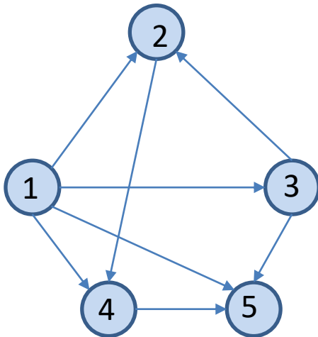
A DAG
